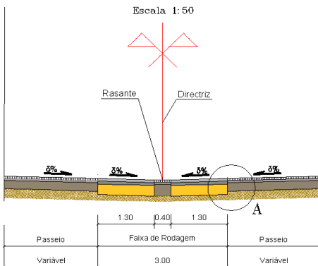
Perfis Transversais Tipo
