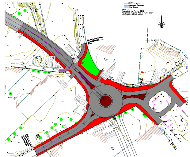
Rotunda do Corvo e ligação à Rua de Sta Catarina
