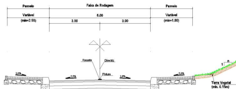
Perfil Transversal Tipo
