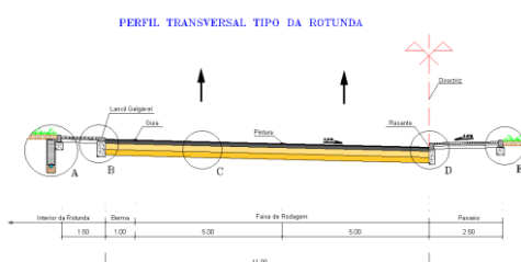
Perfis Transversais Tipo
