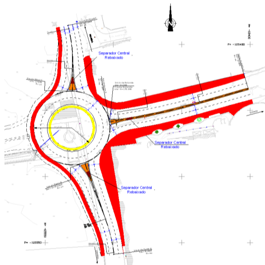
Planta Geral da área de intervenção
