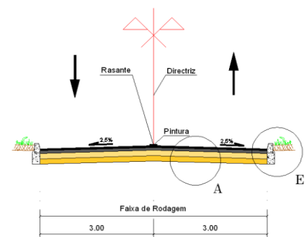
Perfis Transversais Tipo
