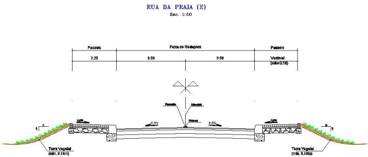
Perfil Transversal Tipo
