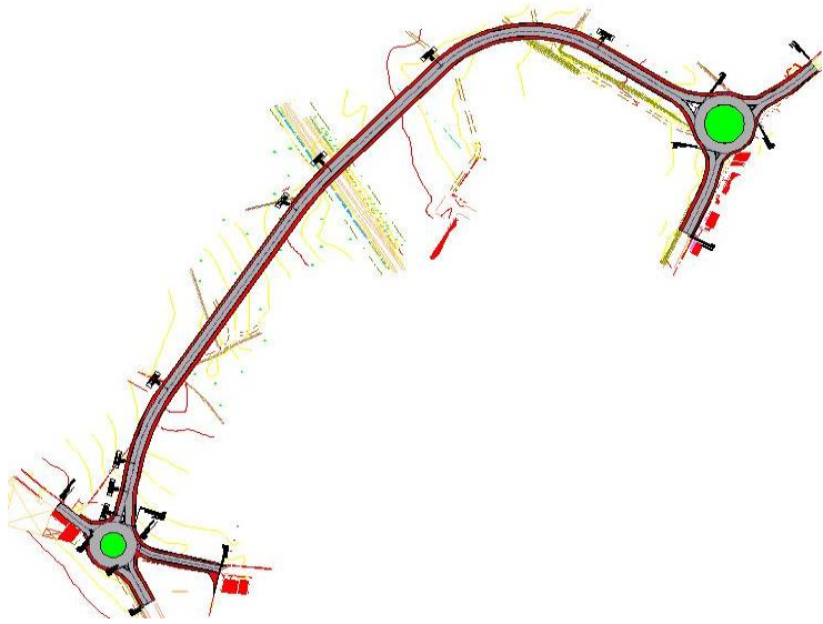
Planta geral da Ligação da Rua da Estação à Variante da Rua da Mota
