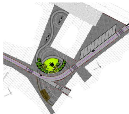
Planta Geral do Traçado
