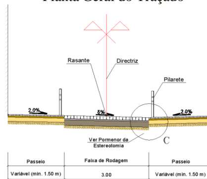
Perfil Transversal Tipo
