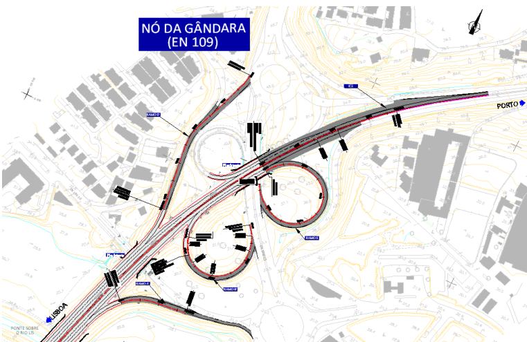
Planta Geral do Nó da Gândara
