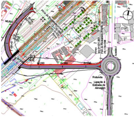
Planta Geral de Traçado do Restabelecimento ao km 116+396
