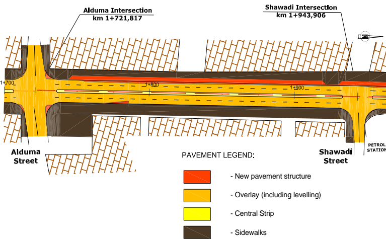
Planta de pavimentação
