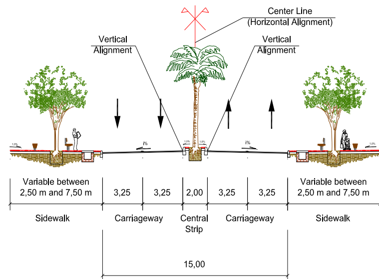
Perfil Transversal Tipo
