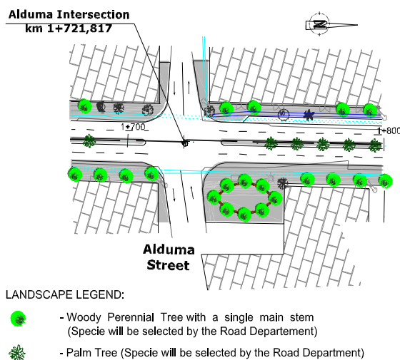
Planta de paisagismo
