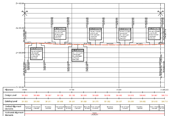
Planta e Perfil Longitudinal da Hospital Street
