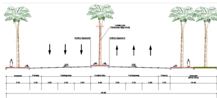
El Nile Street - Perfil Transversal Tipo
