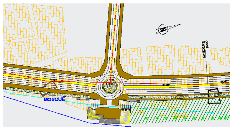
El Nile Street – Intersecção de nível ao km 6+000
