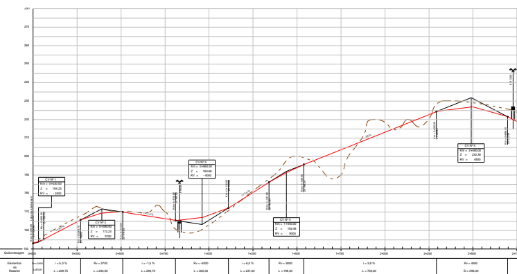
Alternativa A – Perfil Longitudinal
