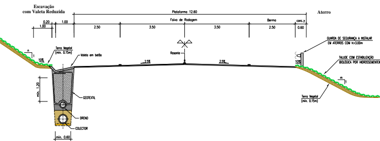
Perfil Transversal Tipo
