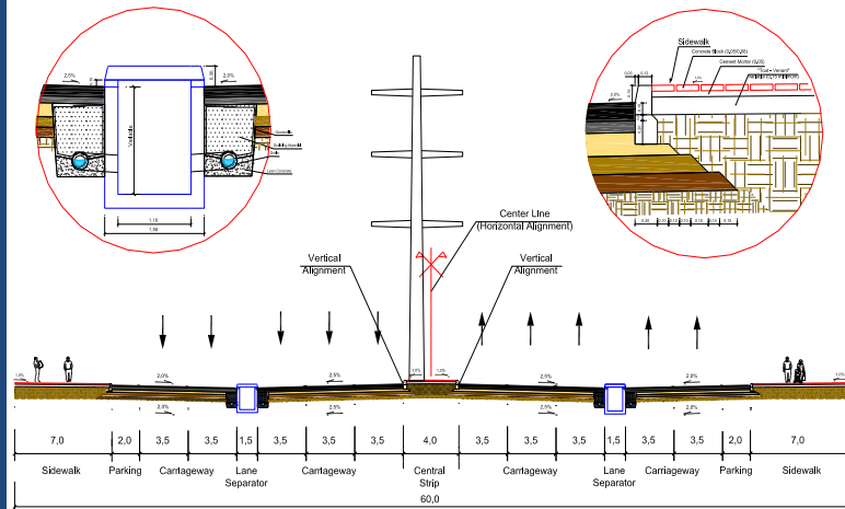
Perfil Transversal Tipo
